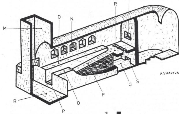
Dibuix esquemàtic ideal del forn de vidre de can Torrella.
