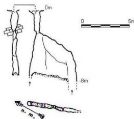
AVENC DE LA CABANA METÀL-LICA Vallirana - Baix Llobregat Topografia: F. Subils - A. Asensio - V. Sans - M. Petronio SEO-CEV
