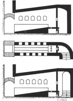
Dibuix esquemàtic ideal del forn de vidre de can Torrella.
