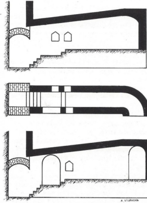
Dibuix esquemàtic actual del forn de vidre matadeperec.
