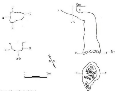
AVENC DEL TRIO Vallirana - Baix Llobregat Topografia: Jordi Esteve (*) EIE - PCB 21 desembre 1989
