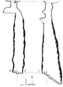
AVENC DE LES RUNES Vallirana - Baix Llobregat Topografia: J. Llonet - J. Marqués SEFOMA
