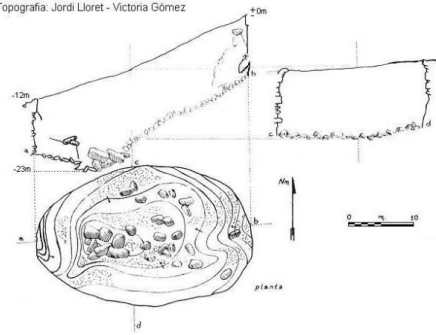
AVENC DE LES PORTES Vallirana - Baix Llobregat Topografia: Jordi Lloret - Victoria Gómez
