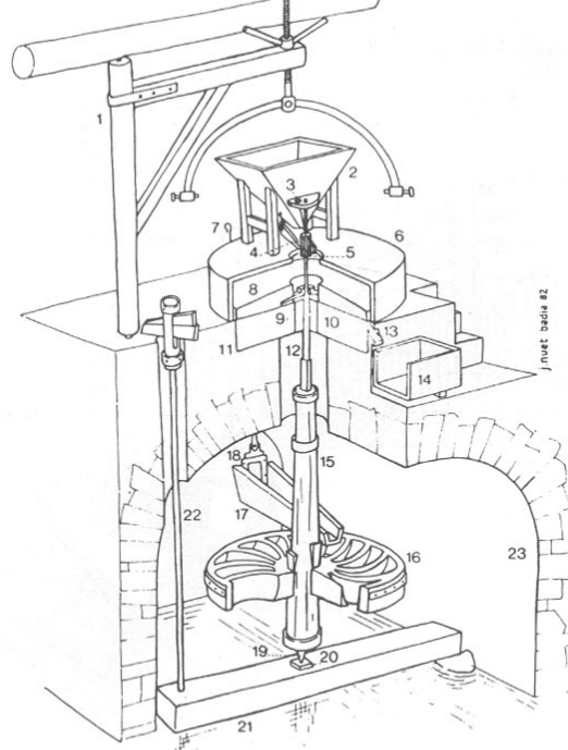
Esquema, tallat un quart, dels mecanismes d'un moli fariner. Les peces principals són: la cabra (1); la tremuja (2); el graduador (3); el canalot (4); la filoseia (5); el riscle (6); l'engegador (7); la mola volandera (8); la nadilla (9); la boixa (10); la mola sotana (11); el coll-ferro (12); el farinal (13); la farineira (14); l'arbre (15); el rodet (16); la canal (17); el pany (18); l'agulla (19); el dau (20); el banc (21); l'alçador (22); el carcabà (23).
